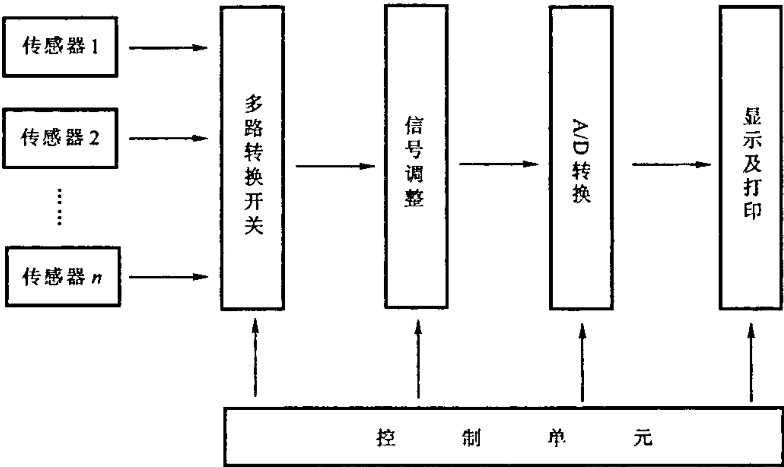
图 1 巡检仪典型结构图
