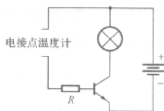
图2 信号电路
